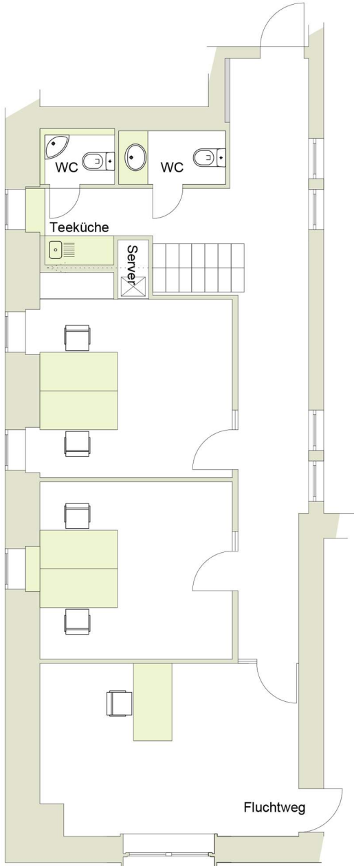
Grundriss Galerie Gartenhaus - 4. OG 1:100
